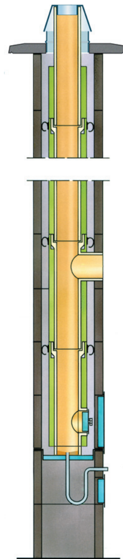
LAS-F Luftabgasschornstein mit Muffenrohr für feste Brennstoffe wie Pellets- und Scheitholzessel
